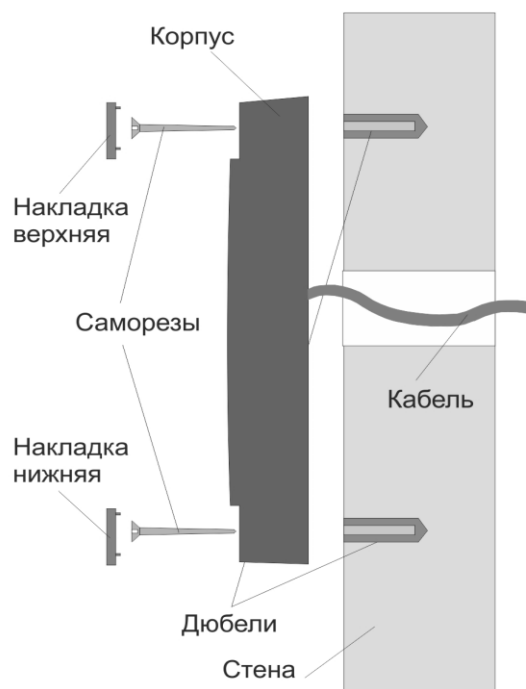
Рисунок 2. Крепление считывателя
