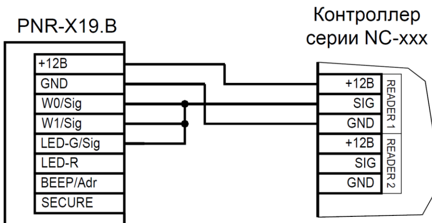
Рисунок 5. Подключение считывателя в режиме Parsec, адрес 1 (внутренний)
